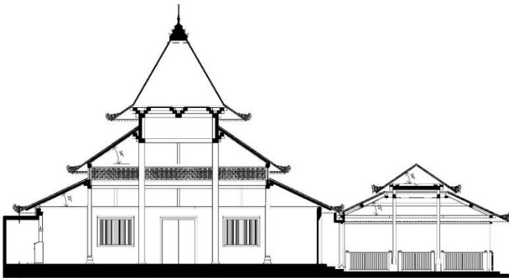
Gambar potongan masjid
