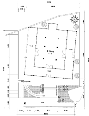
Gambar siteplan rencana awal masjid tanpa serambi
