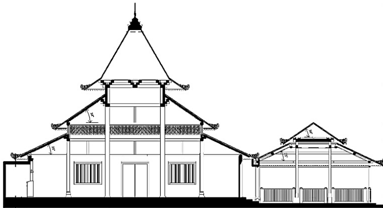
Gambar Potongan Masjid Ki Mageti
