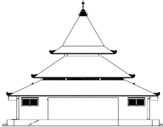
1 TAMPAK BARAT A04 Scale: 1 : 100
