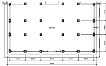
1 DENAH SERAMBI A01 Scale: 1 : 100
